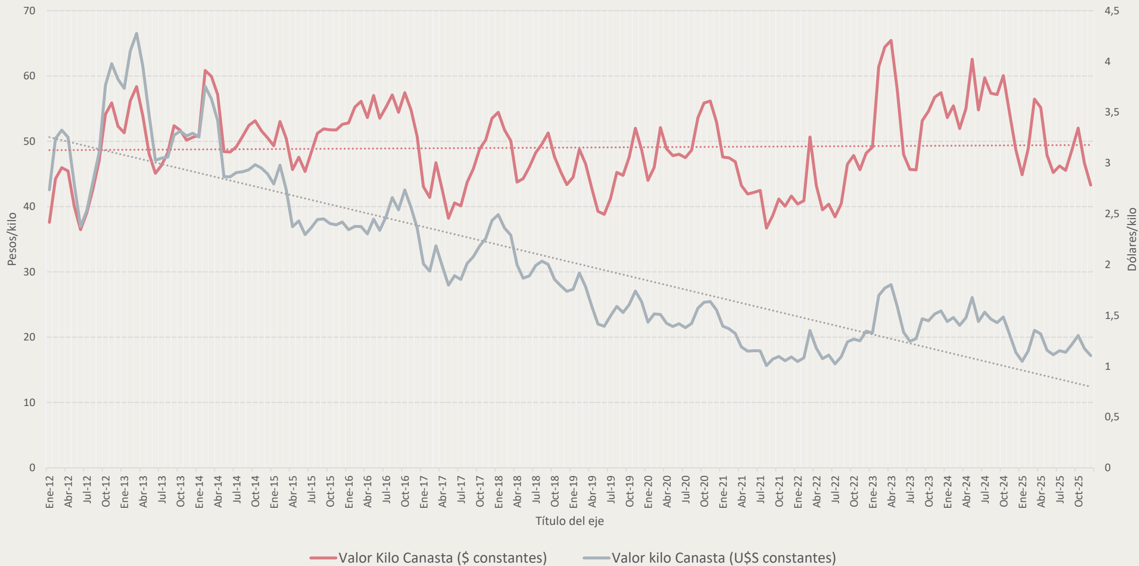
Evolución mensual del VKC en pesos constantes y en dólares estadounidenses, ambos corregidos a diciembre de 2025
